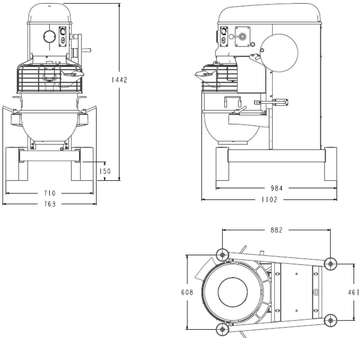
ABBILDUNG 5 H800S SCHIFFSVERSION PLANETENRÜHRMASCHINE GESAMTABMESSUNGEN (BEFESTIGUNGSNABE OPTIONAL).
