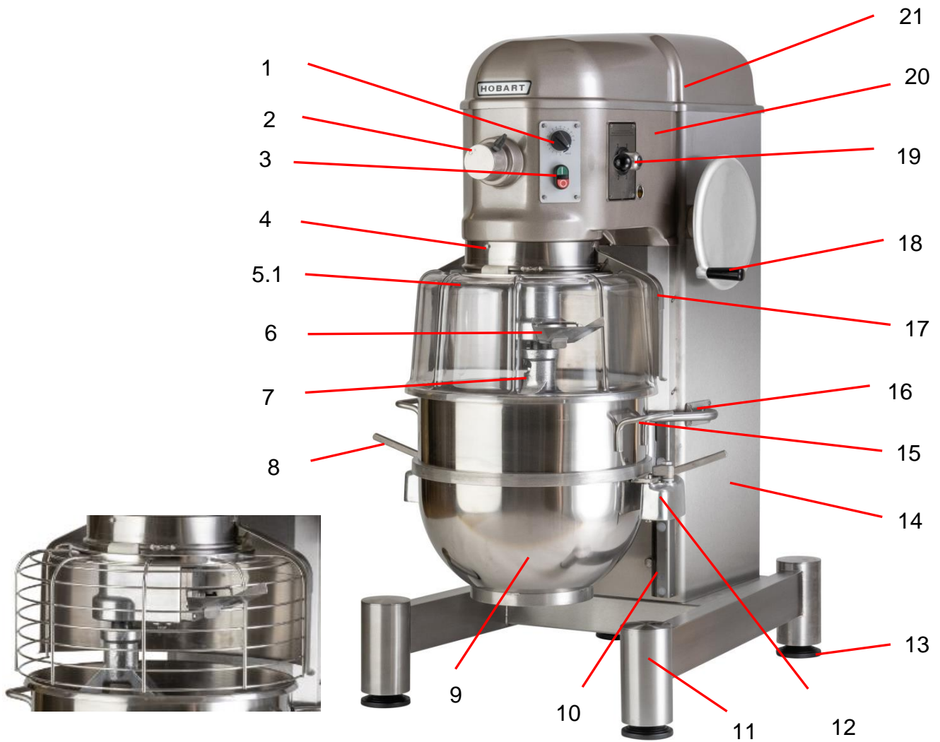
FIGURE 1. IDENTIFICACIÓN DE LOS COMPONENTES DE LA MEZCLADORA
