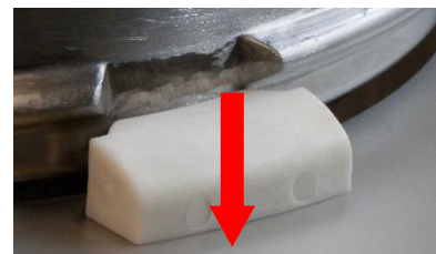
6. Continuer à faire tourner le pare-poussière jusqu'à ce que le bloc de guidage blanc soit aligné sur la découpe située au bord de la coupelle.
