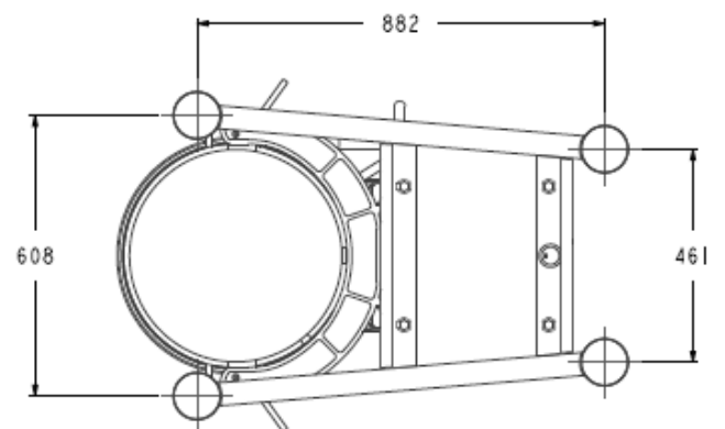
ABBILDUNG 2 H600S STANDARDVERSION PLANETENRÜHRMASCHINE GESAMTABMESSUNGEN (BEFESTIGUNGSNABE OPTIONAL)
