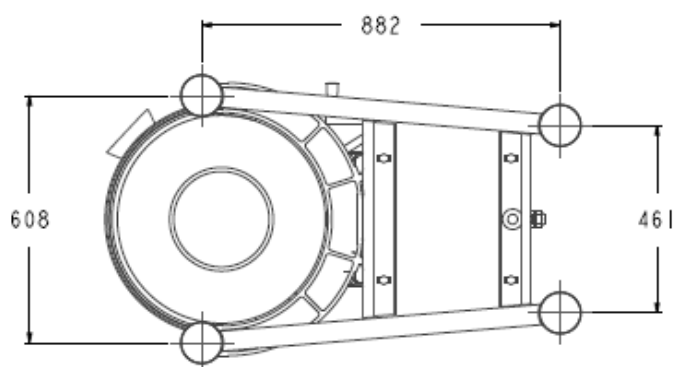
FIGURE 4. DIMENSIONS HORS TOUT DU BATTEUR MÉLANGEUR ALIMENTAIRE STANDARD H800S (MOYEU DE FIXATION DES ACCESSOIRES EN OPTION).
