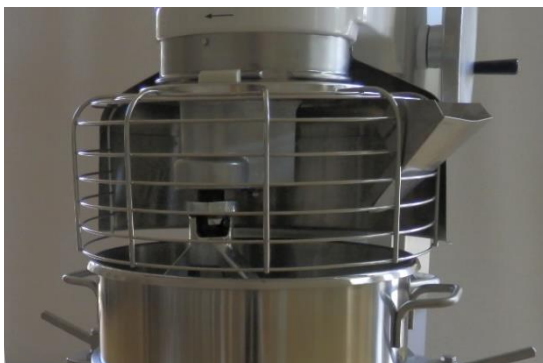
2. Cage de protection métallique fermée et goulotte de versement des ingrédients installée.
