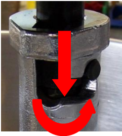
5. Retirer le malaxeur en tournant dans le sens anti-horaire et en tirant vers le bas.
