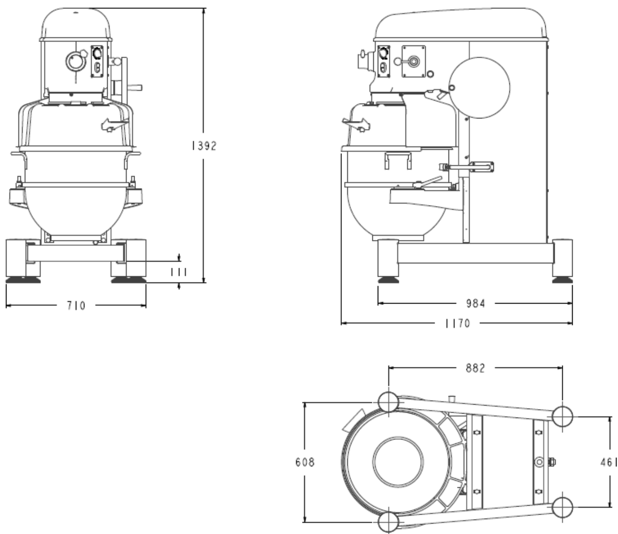
FIGURA 4: DIMENSIONES TOTALES DE MEZCLADORA PLANETARIA H800S MODELO ESTÁNDAR (PORTAACCESORIOS OPCIONAL)
