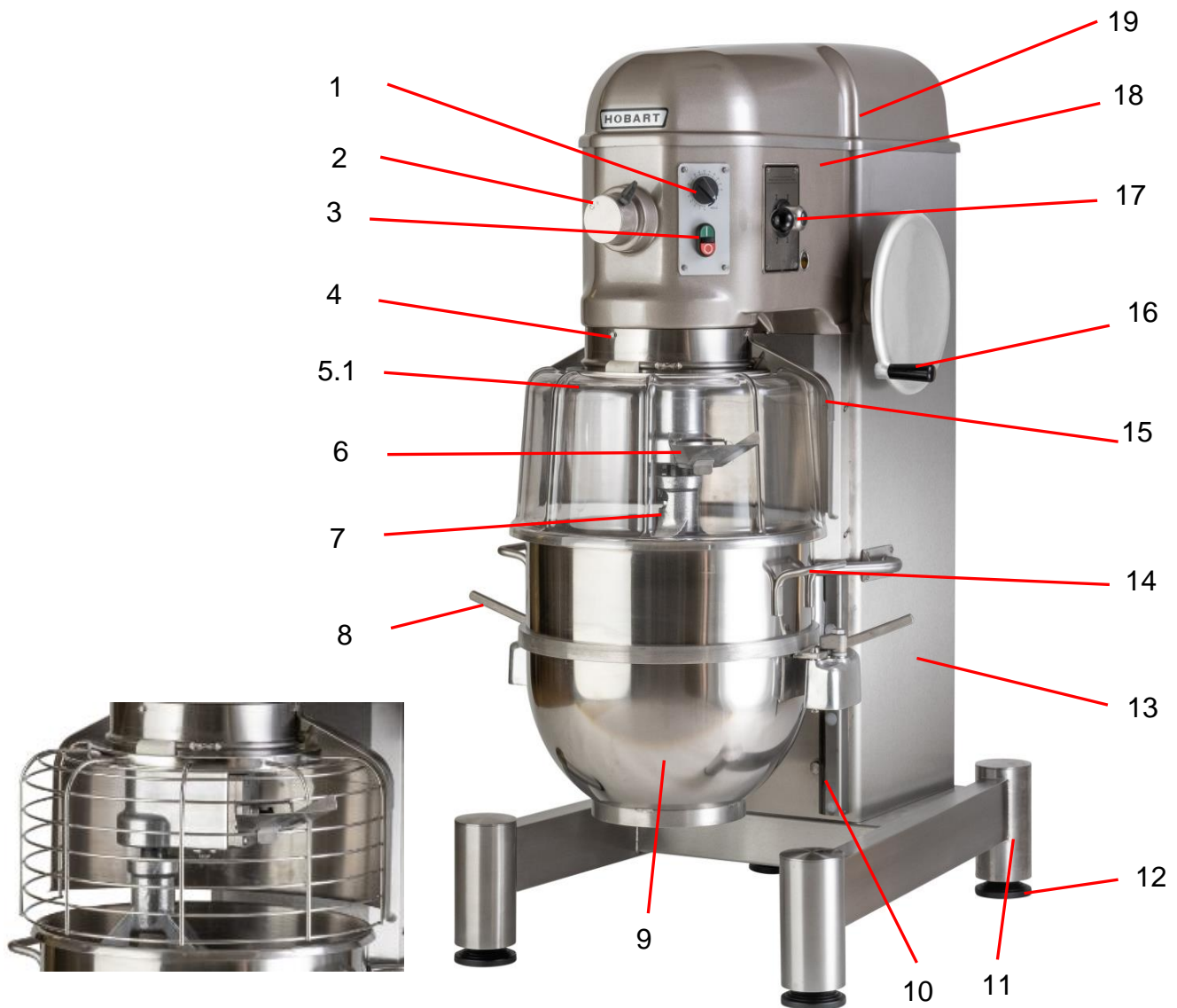
5.2 FIGURE 1. IDENTIFICATION DES COMPOSANTS DU MÉLANGEUR.
