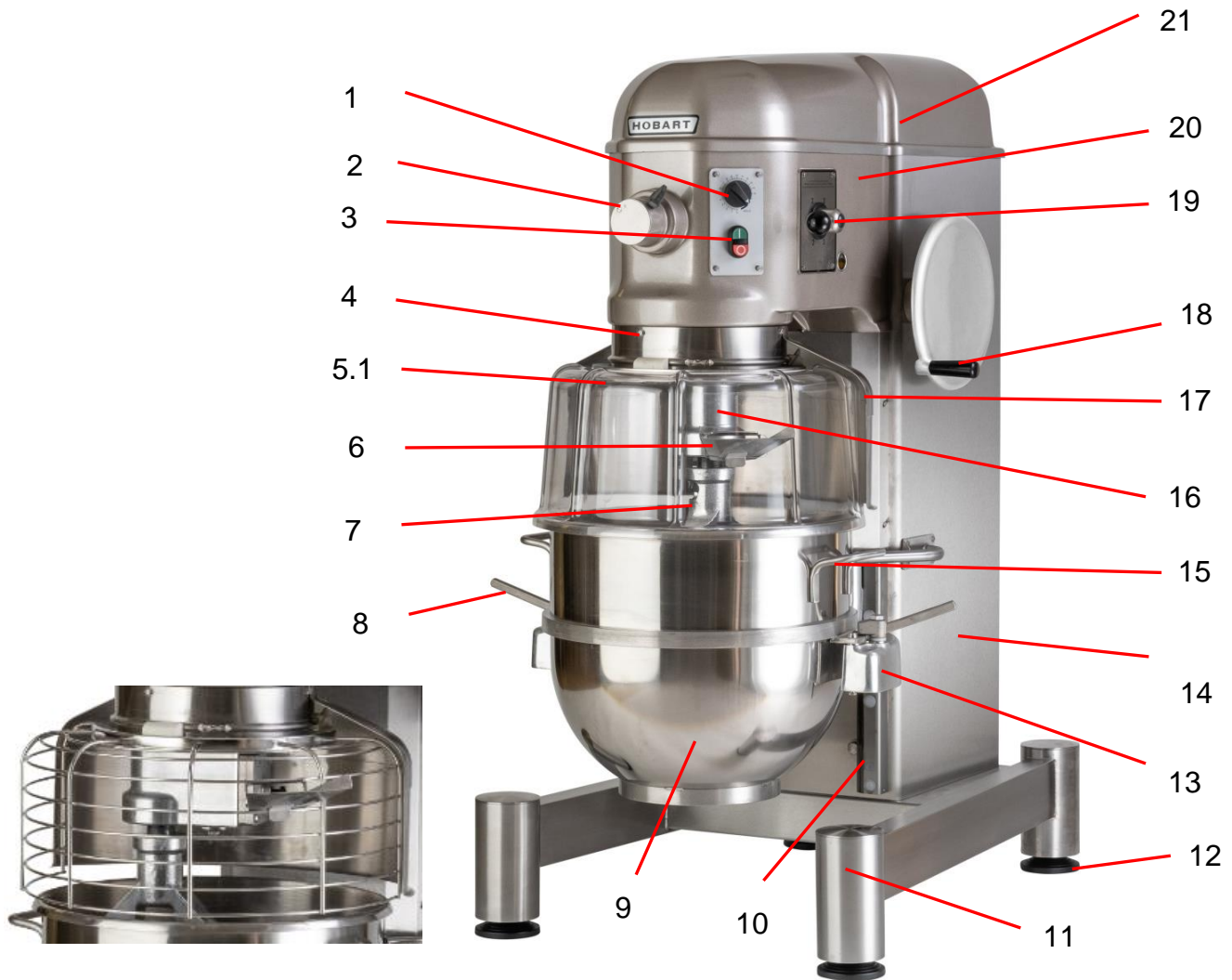
ABBILDUNG 1 BESTANDTEILE DER RÜHRMASCHINE
