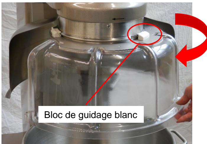
6. Continuer à faire tourner le pare-poussière jusqu'à ce que le bloc de guidage blanc soit aligné sur la découpe située au bord de la coupelle.
