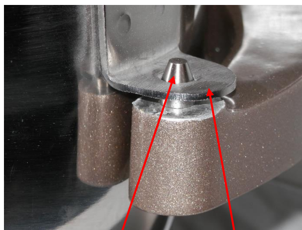
Ergot du bol et goupille de positionnement
