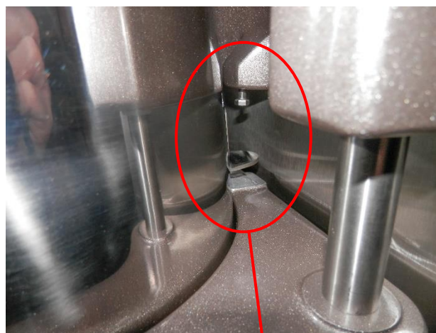
Butée arrière du bol et ergot du bol
