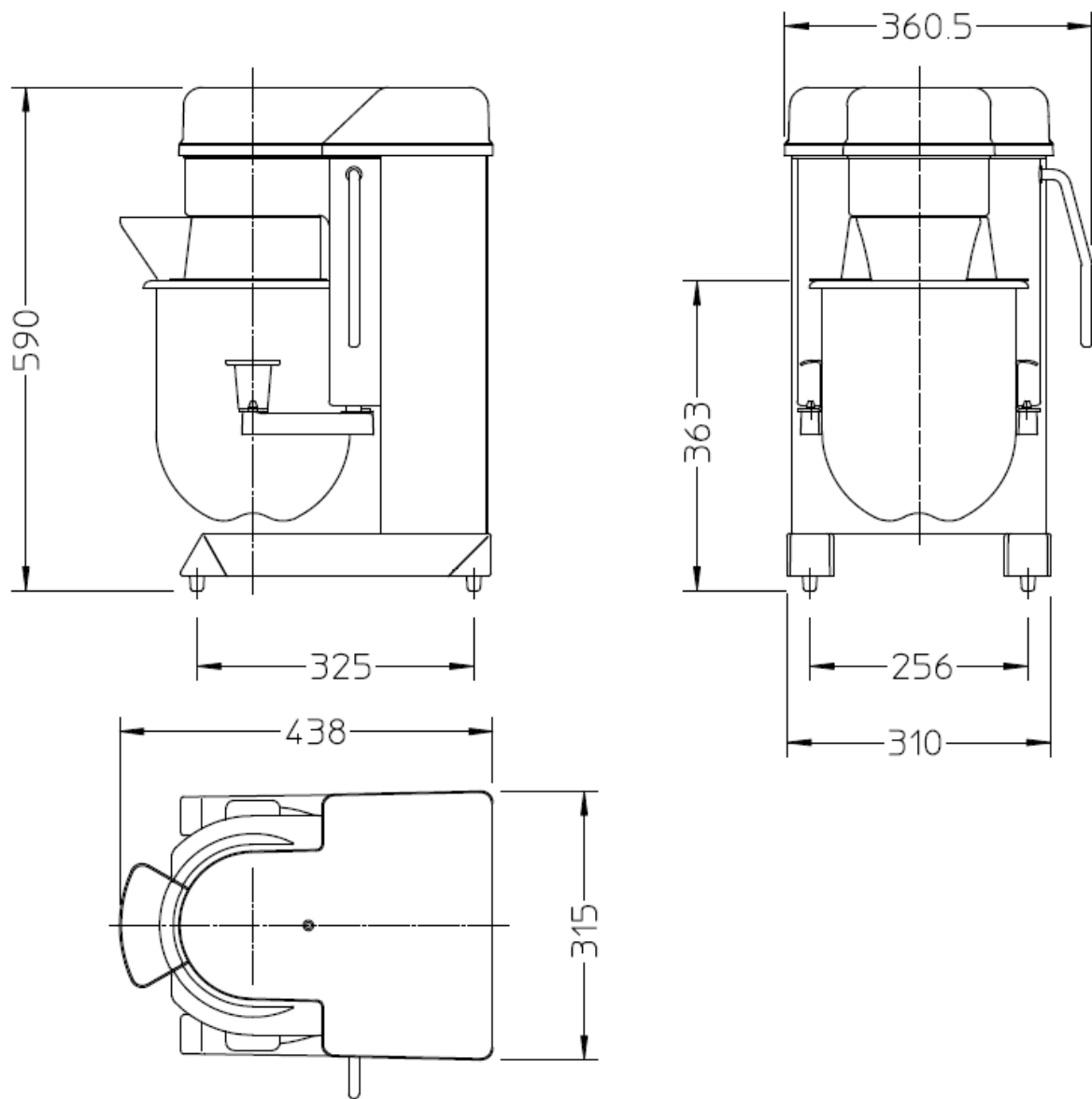
FIGURE 2. DIMENSIONS HORS TOUT DU BATTEUR MÉLANGEUR ALIMENTAIRE HSM10N
