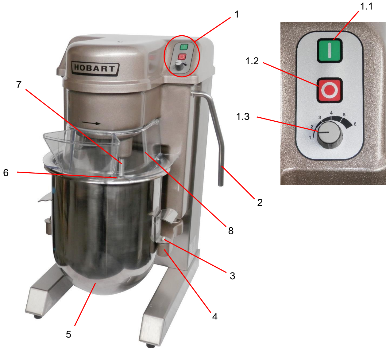
ABBILDUNG 1 BESTANDTEILE DER RÜHRMASCHINE
