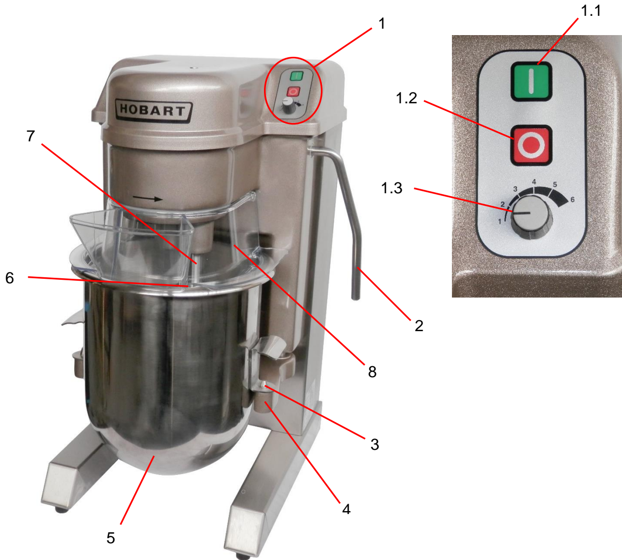
FIGURE 1. IDENTIFICACIÓN DE LOS COMPONENTES DE LA MEZCLADORA
