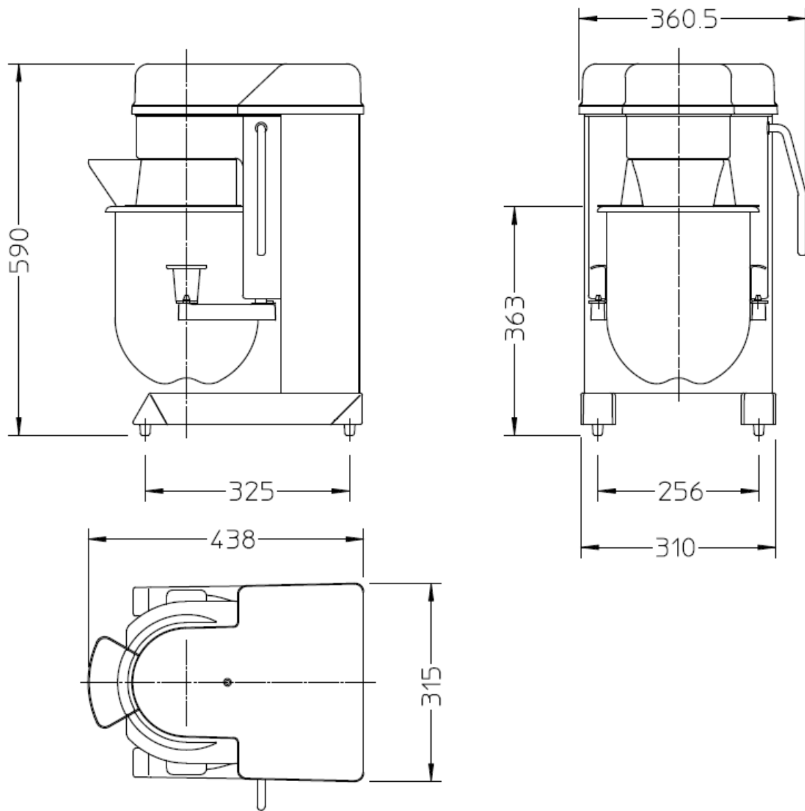
FIGURA 2. HSM10N DIMENSIONES TOTALES DE MEZCLADORA PLANETARIA
