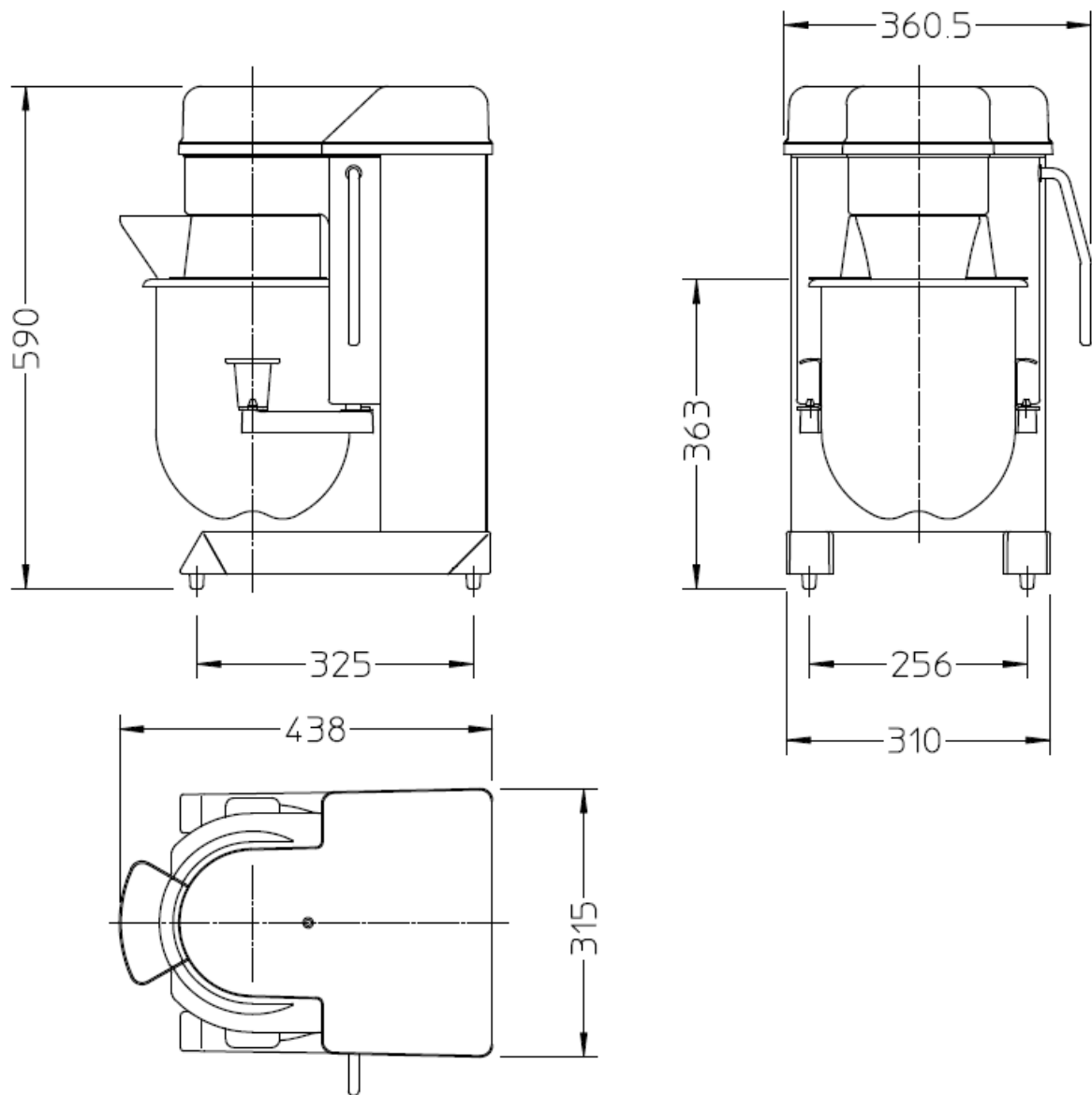
FIGURE 2. HSM10N PLANETENRÜHRMASCHINE GESAMTABMESSUNGEN
