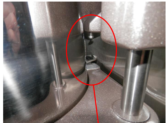
Hinterer Kesselanschlag und Kesselzapfen
