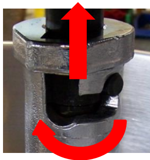
Saliente del recipiente y espiga de posicionamiento
