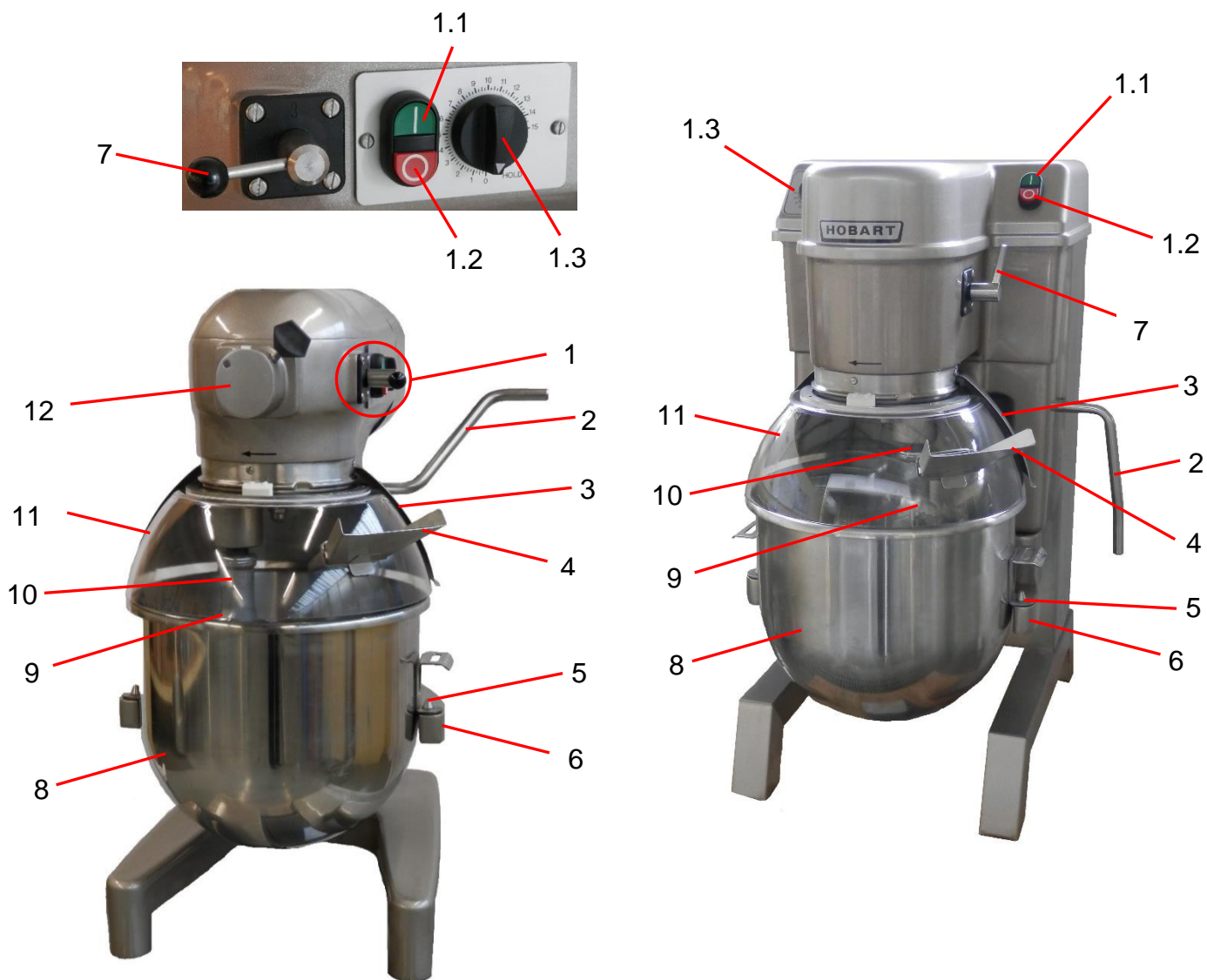
FIGURA 1. IDENTIFICACIÓN DE LOS COMPONENTES DE LA MEZCLADORA
