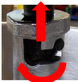
Ergot du bol et goupille de positionnement
