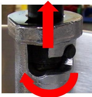
Kesselzapfen und Positionierstift
