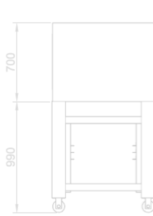
VISTA POSTERIORE + SUPPORTO BACK VIEW + STAND
